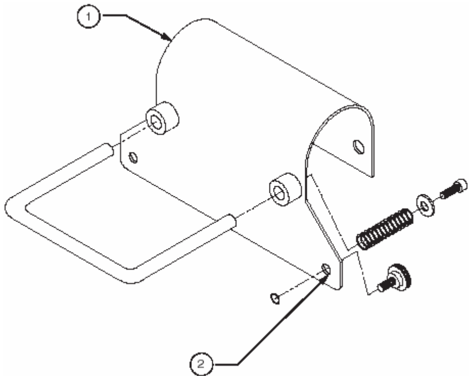
图 3 人孔横档悬架
